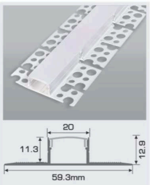
B20 - 2 D W59.3 x H12.9mm 256.000/m Nhôm định hình + Chụp nhựa Dẻo
