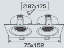
AFC 391 T/2 - MR16 (Không Bóng) 361.000
