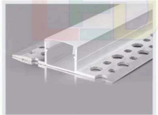
A15 - 2 D W55.3 x H12.8mm 156.000/m Nhôm định hình + Chụp nhựa PC
