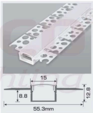
B15 - 2 T W55.3 x H12.8mm 236.000/m Nhôm định hình + Chụp nhựa Dẻo
