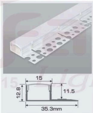
B15 - 1 D W35.3 x H12.8mm 216.000/m Nhôm định hình + Chụp nhựa Dẻo
