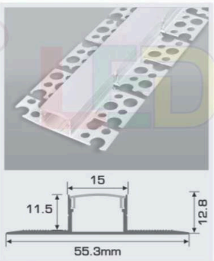
B15 - 2 D W55.3 x H12.8mm 236.000/m Nhôm định hình + Chụp nhựa Dẻo
