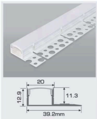
B20 - 1 D W39.2 x H12.9mm 236.000/m Nhôm định hình + Chụp nhựa Dẻo
