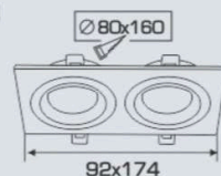
AFC 388 T/2 - MR16 (Không Bóng) 464.000
