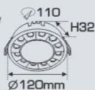
AFC 664 LED 12W 3 chức năng sáng 628.000
