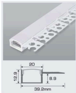
B20 - 1 T W39.2 x H12.9mm 236.000/m Nhôm định hình + Chụp nhựa Dẻo
