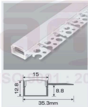
B15 - 1 T W35.3 x H12.8mm 216.000/m Nhôm định hình + Chụp nhựa Dẻo
