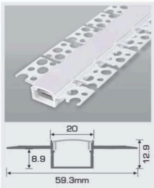
B20 - 2 T W59.3 x H12.9mm 256.000/m Nhôm định hình + Chụp nhựa Dẻo
